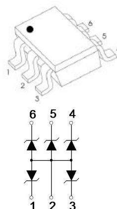
SOT-363
